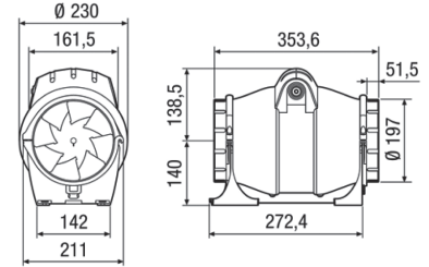
AXM 200
