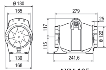
AXM 125
